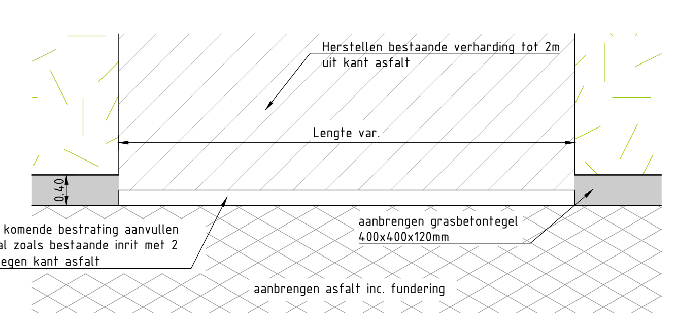
Principedetail verharde inrit Schaal 1:50
