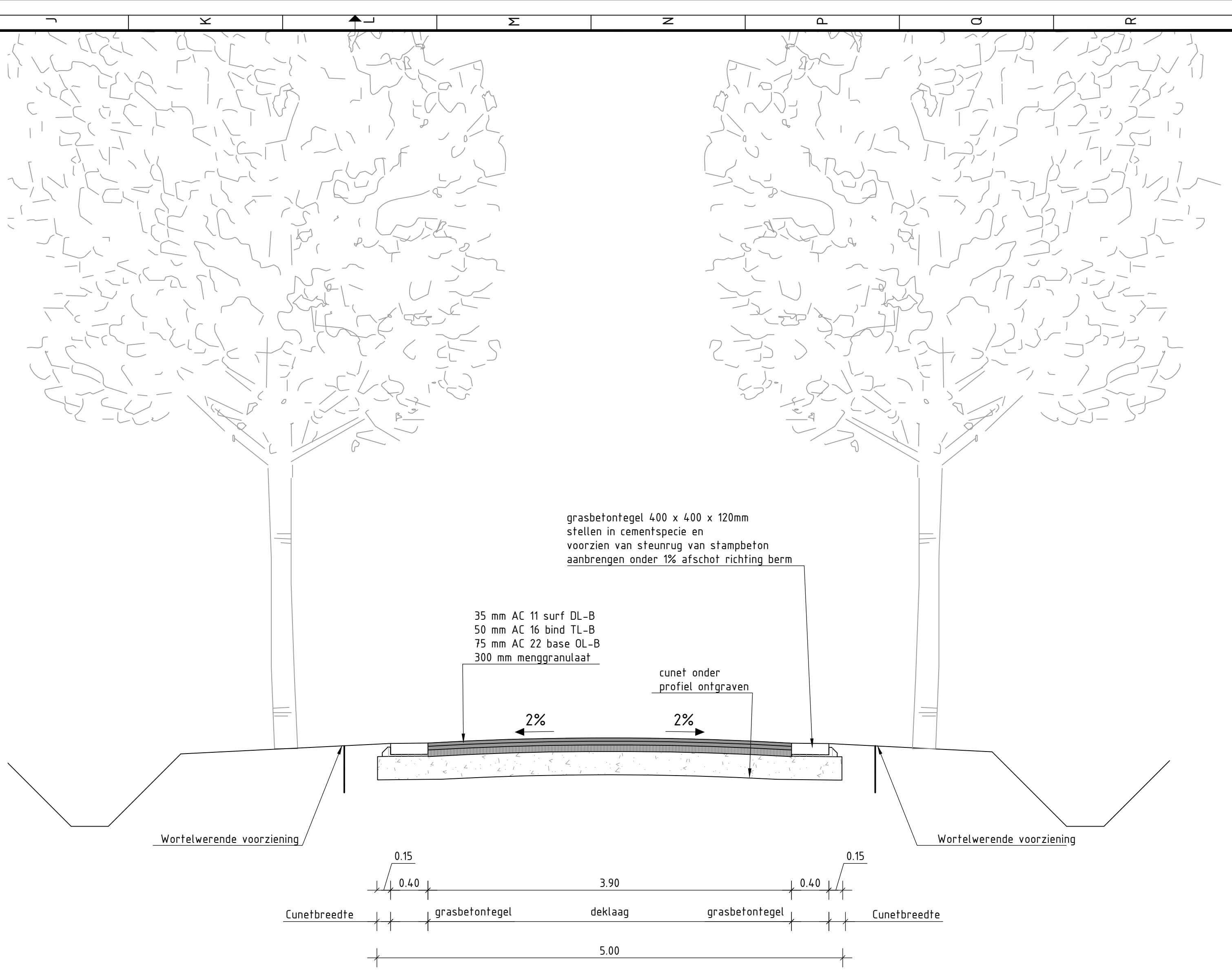
Principe doorsnede Schaal 1:50
